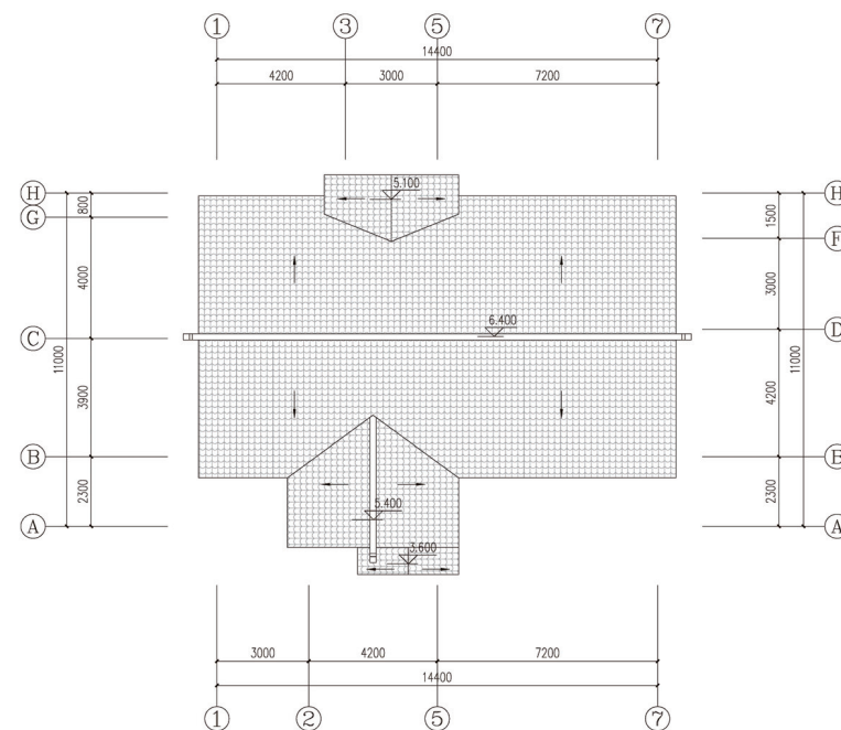
屋顶层平面图
