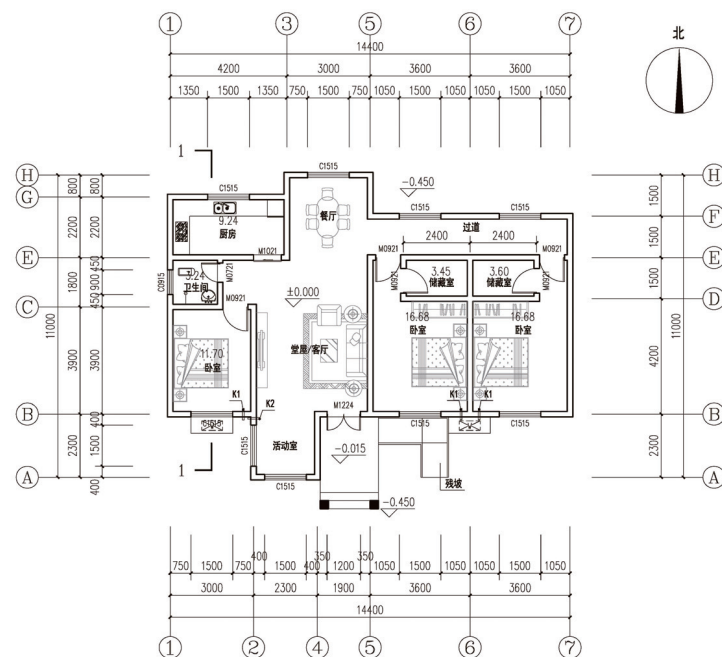
一层平面图
