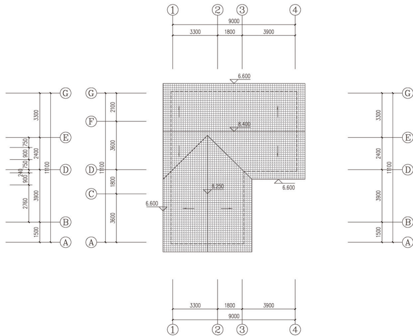
屋顶层平面图
