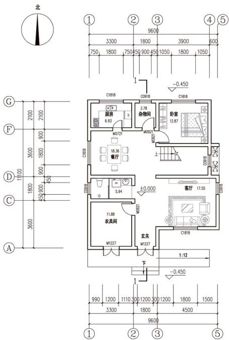
一层平面图
