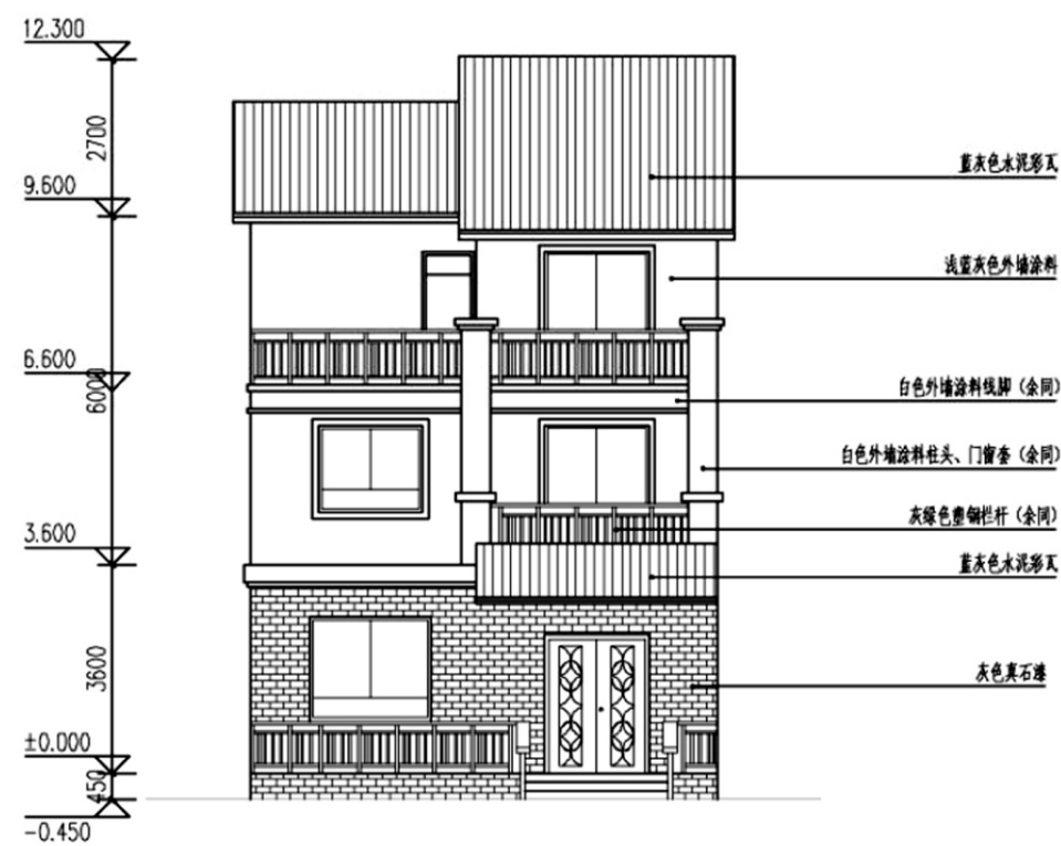
南立面图
