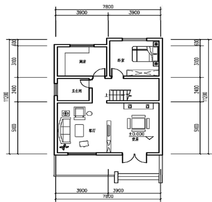
一层平面图
