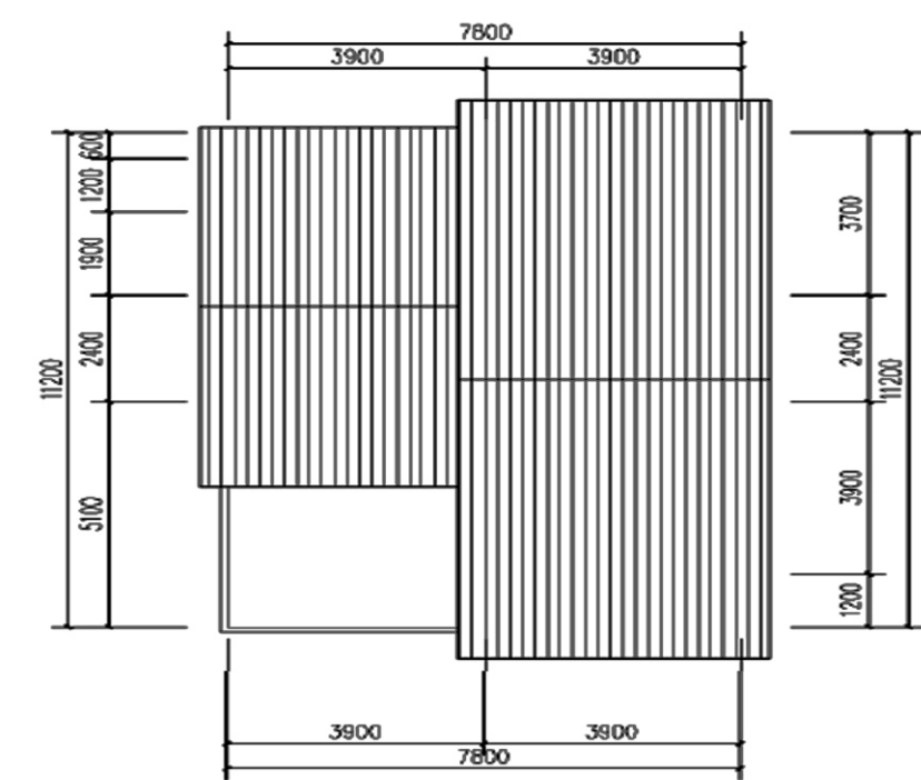
二层平面图
