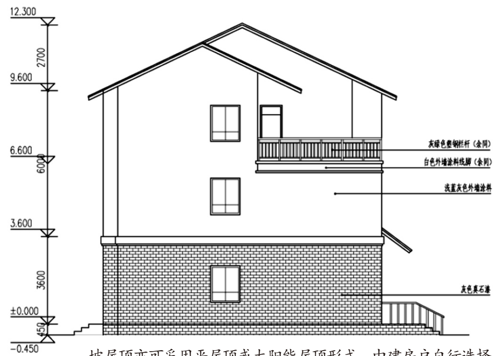
西立面图
