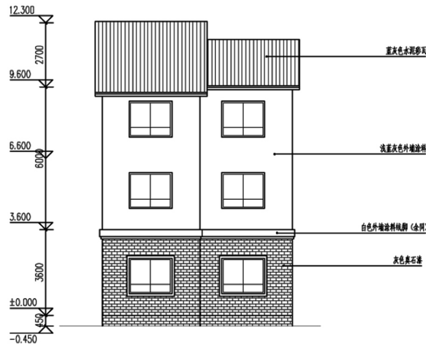
北立面图
