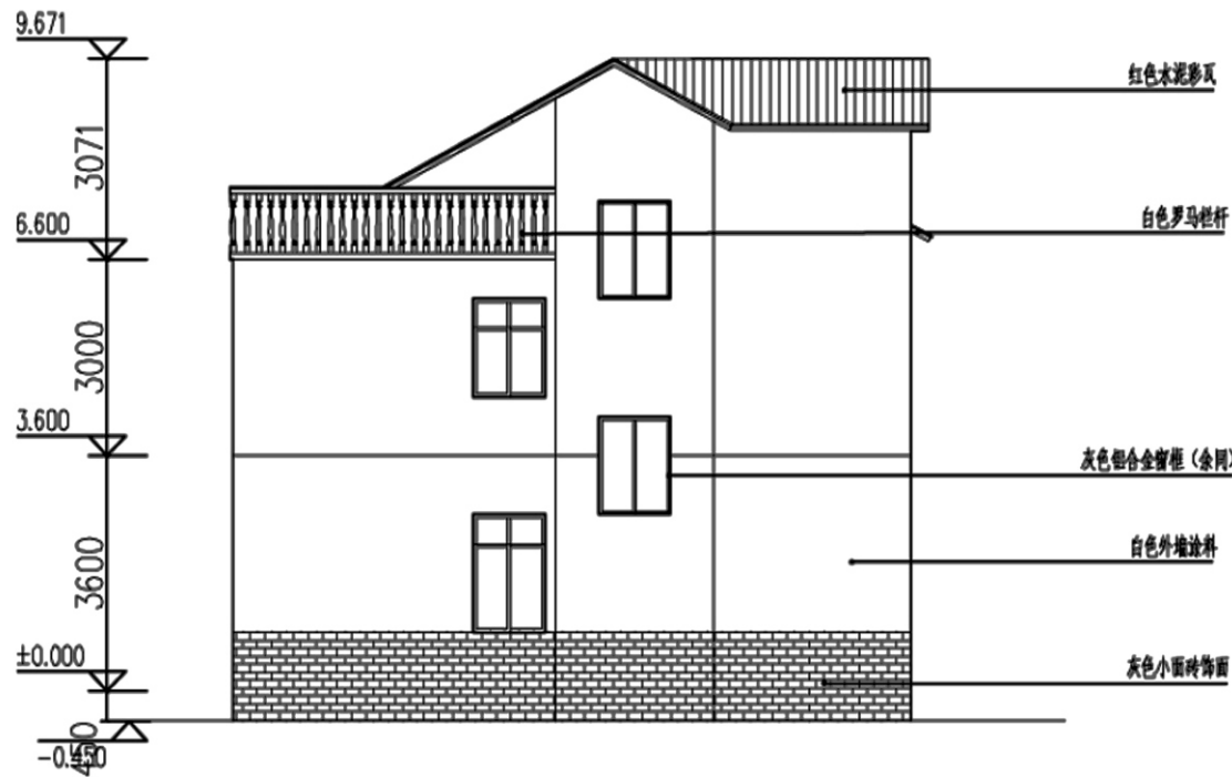
东立面图
