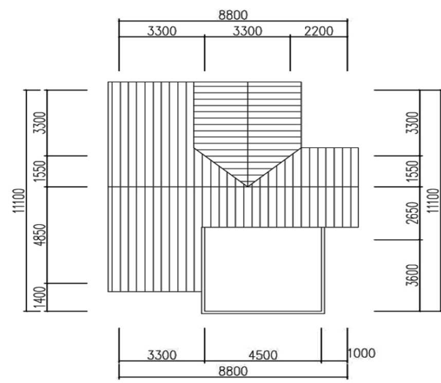
屋顶平面图
