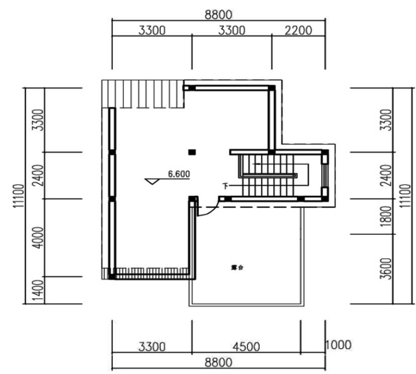
阁楼平面图
