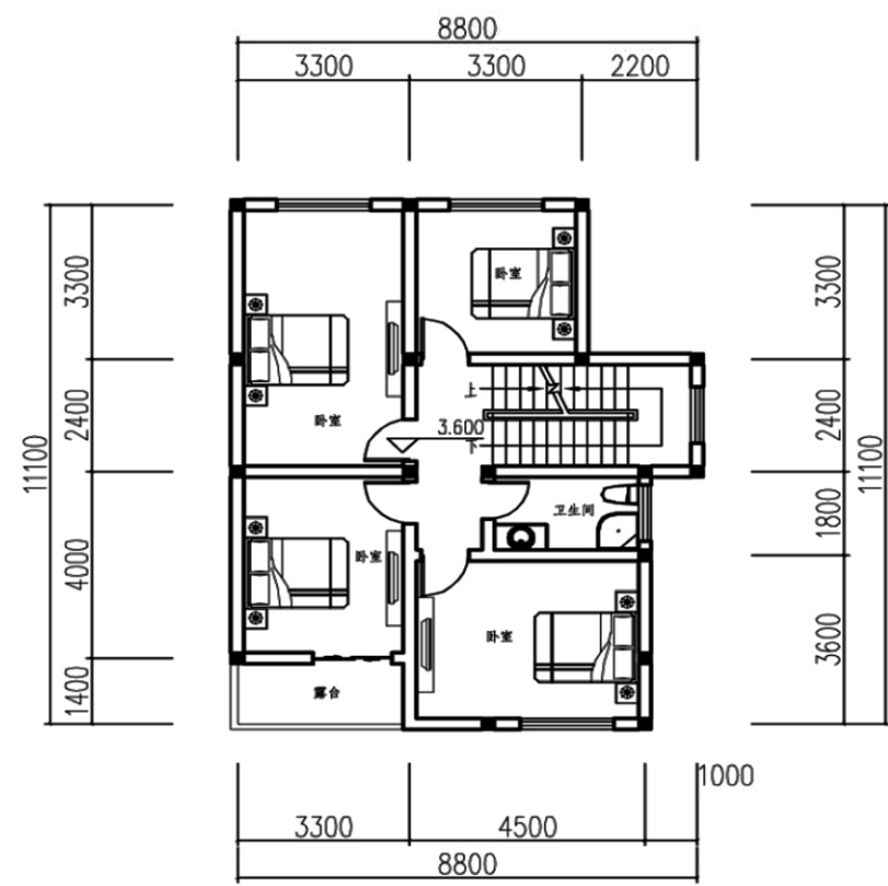
二层平面图
