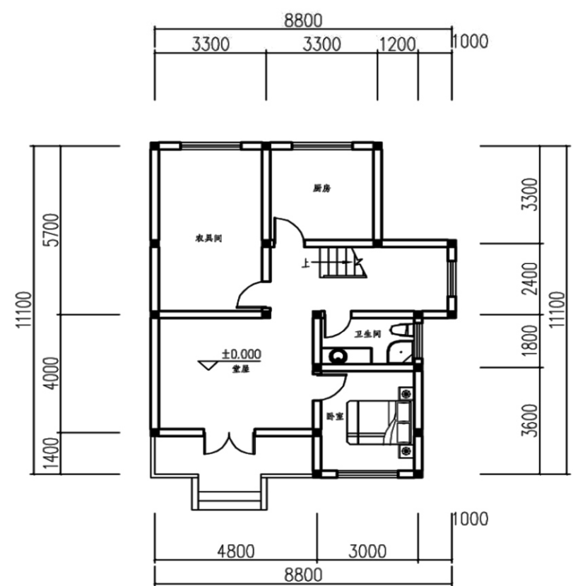
一层平面图
