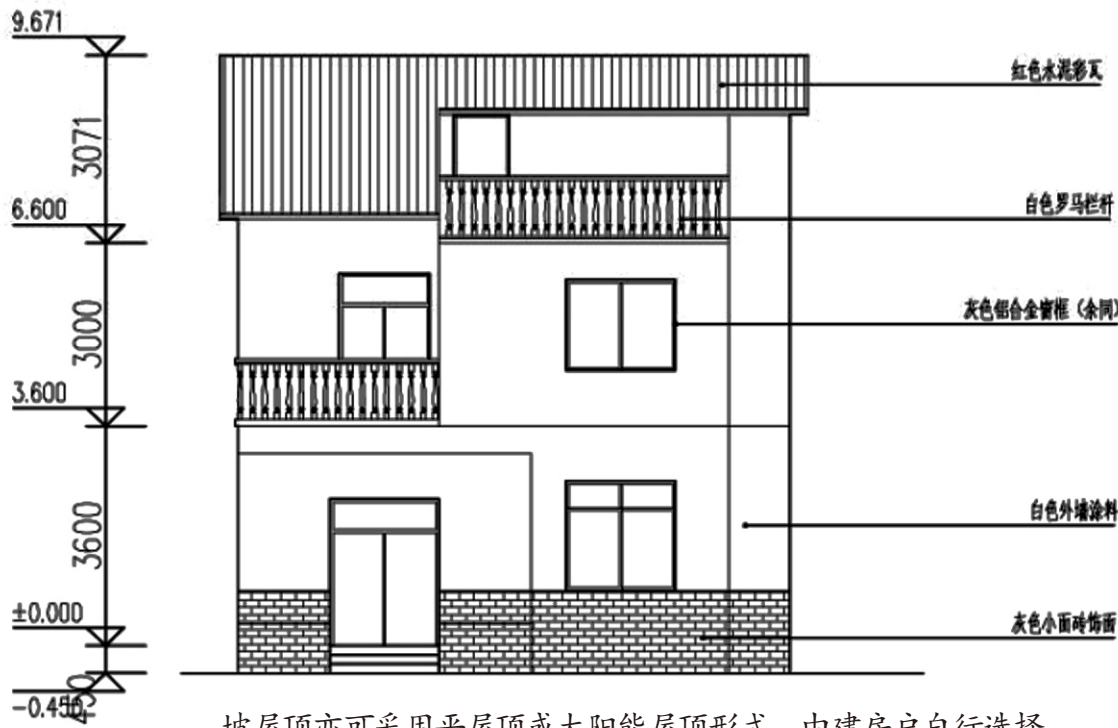
南立面图
