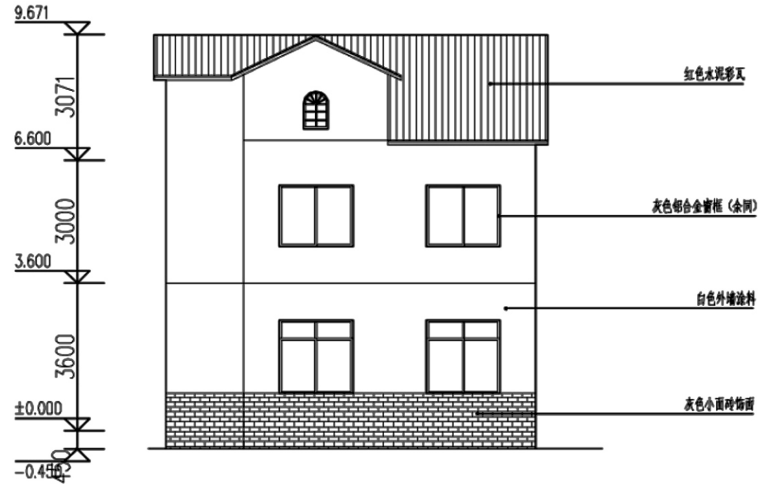
北立面图
