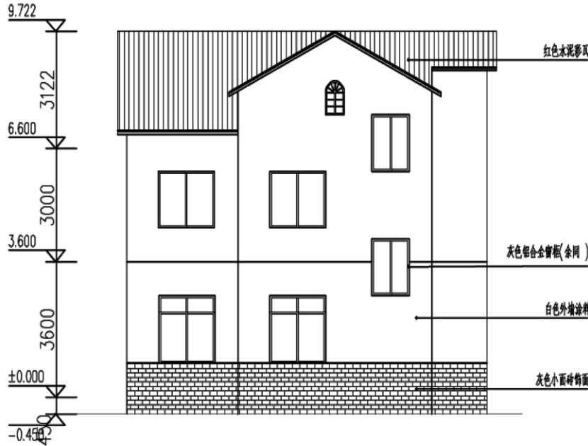
北立面图
