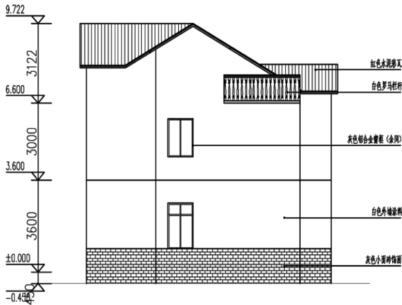
西立面图
