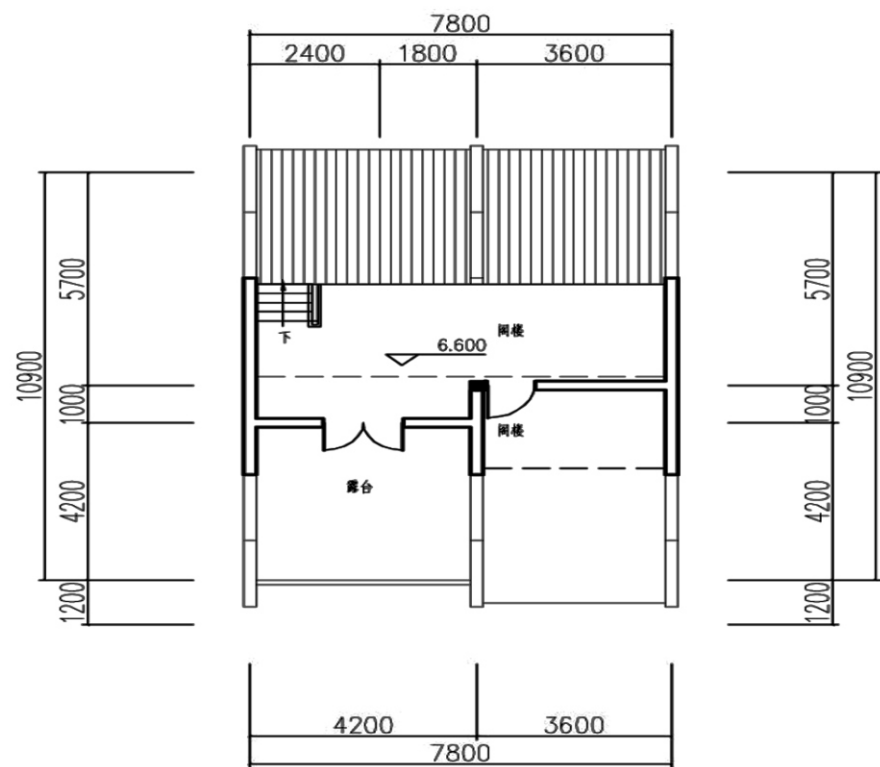
阁楼平面图
