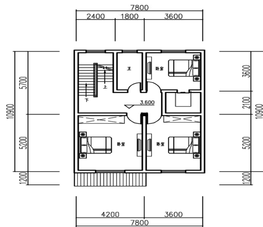
二层平面图
