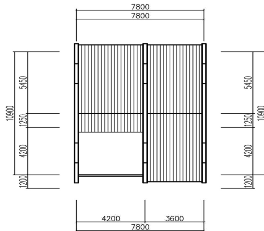
屋顶平面图
