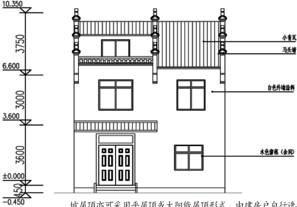
正立面图
