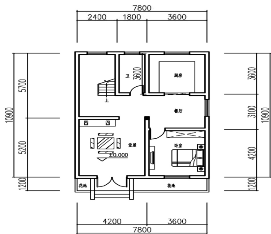
一层平面图
