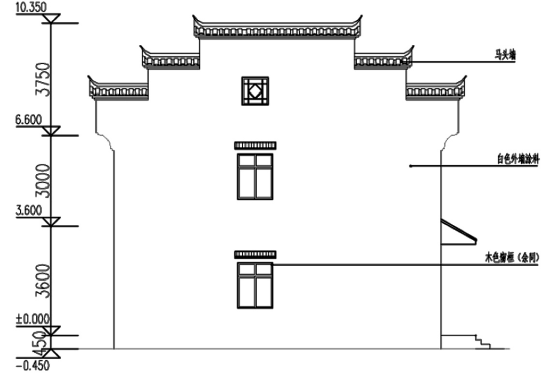
侧立面图
