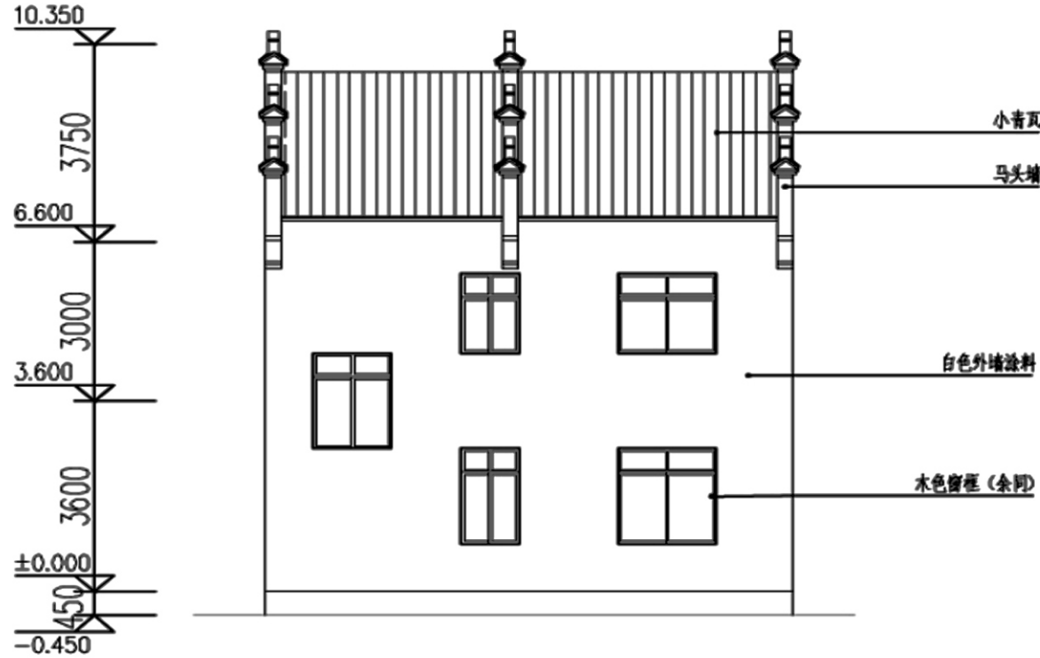
背立面图
