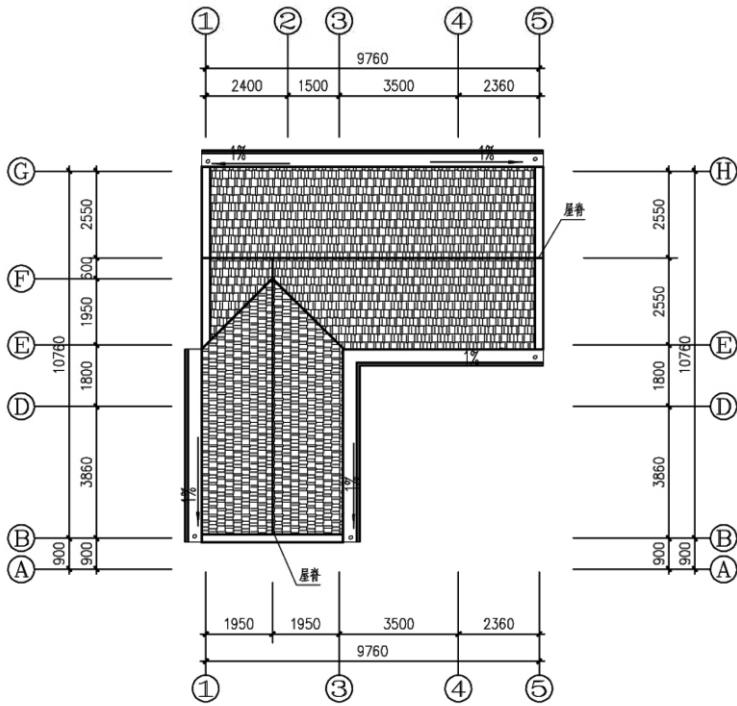
屋顶平面图
