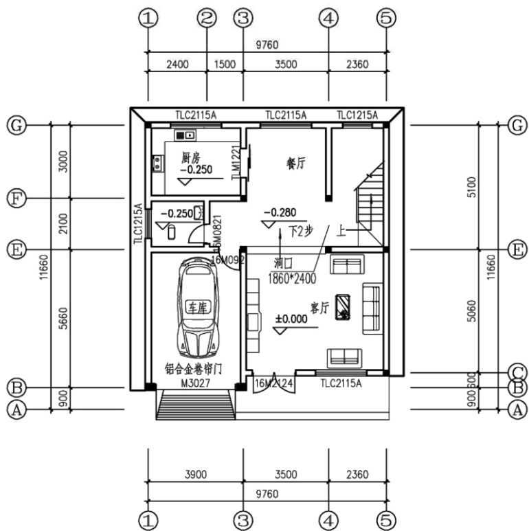
一层平面图
