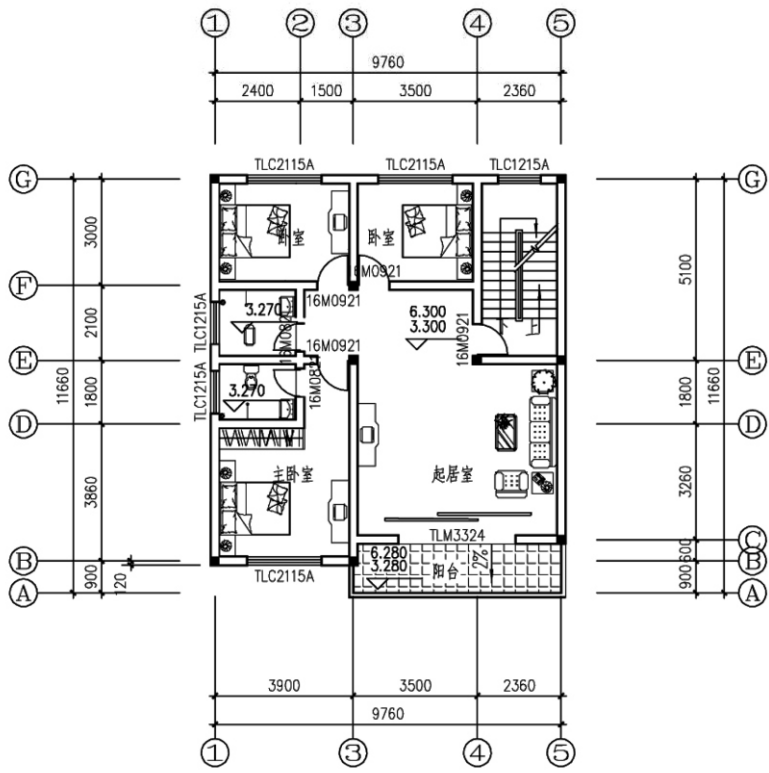
二~三层平面图
