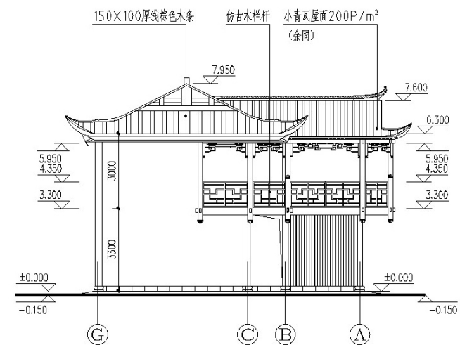
西立面图
