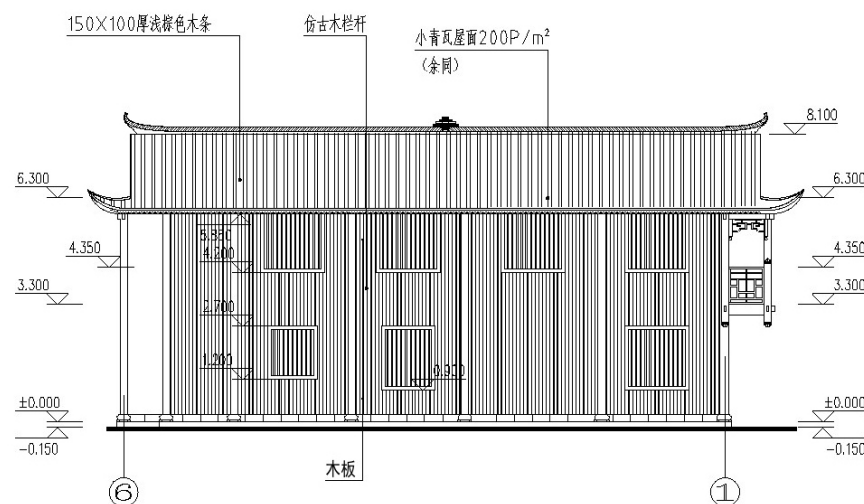
北立面图
