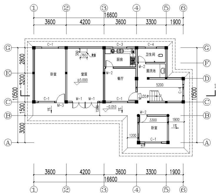
一层平面图
