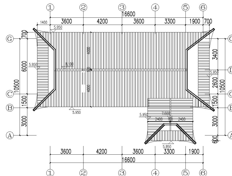
屋顶平面
