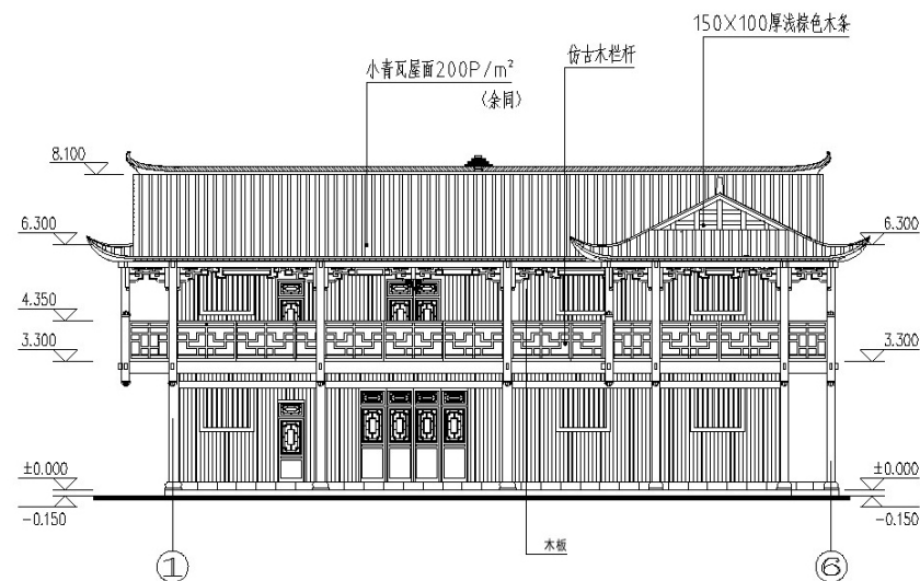
南立面图
