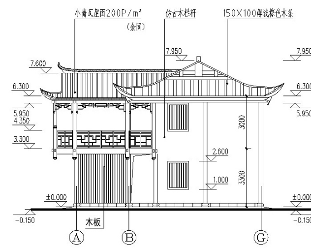
东立面图
