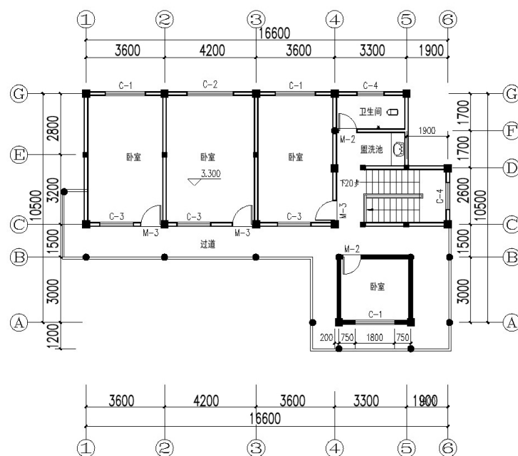
二层平面图
