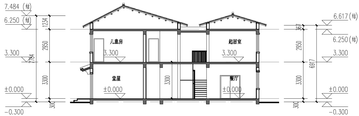
剖面图
