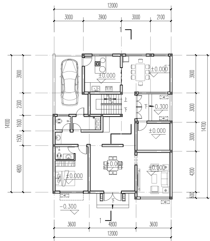
一层平面图
