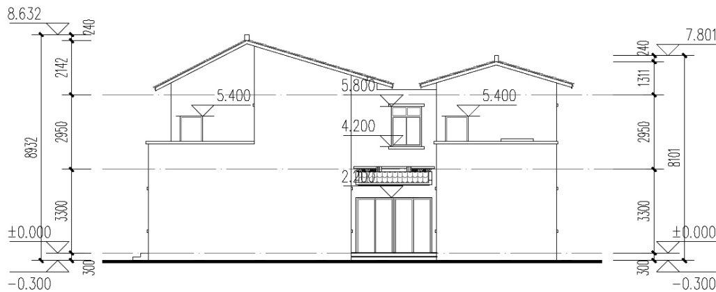
东立面图
