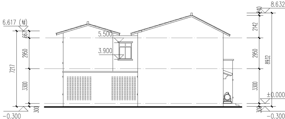
西立面图
