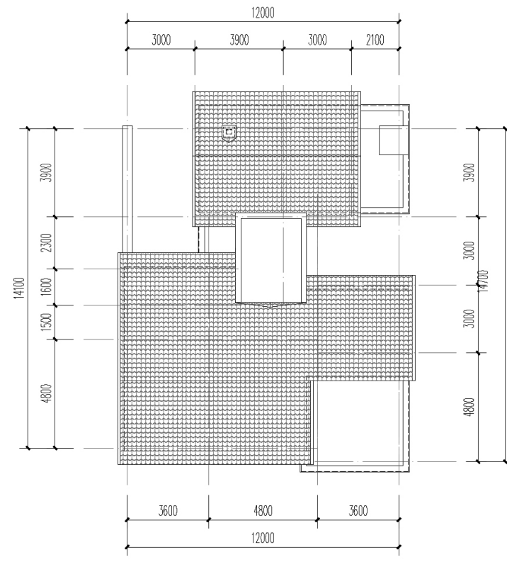
屋顶平面
