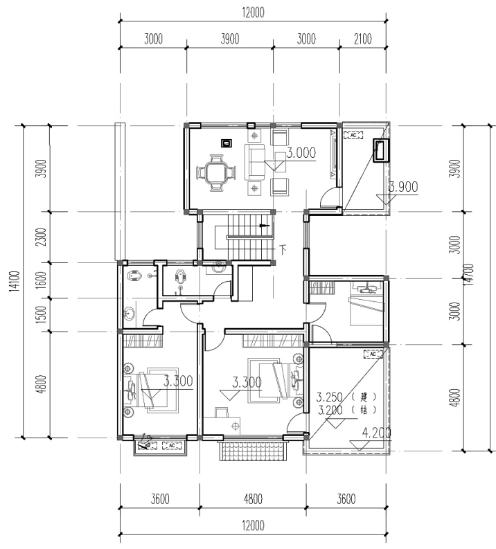
二层平面图
