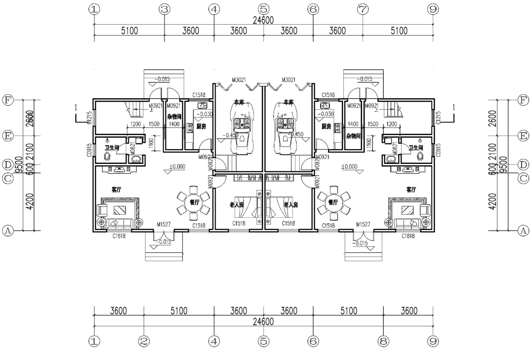
一层平面图
