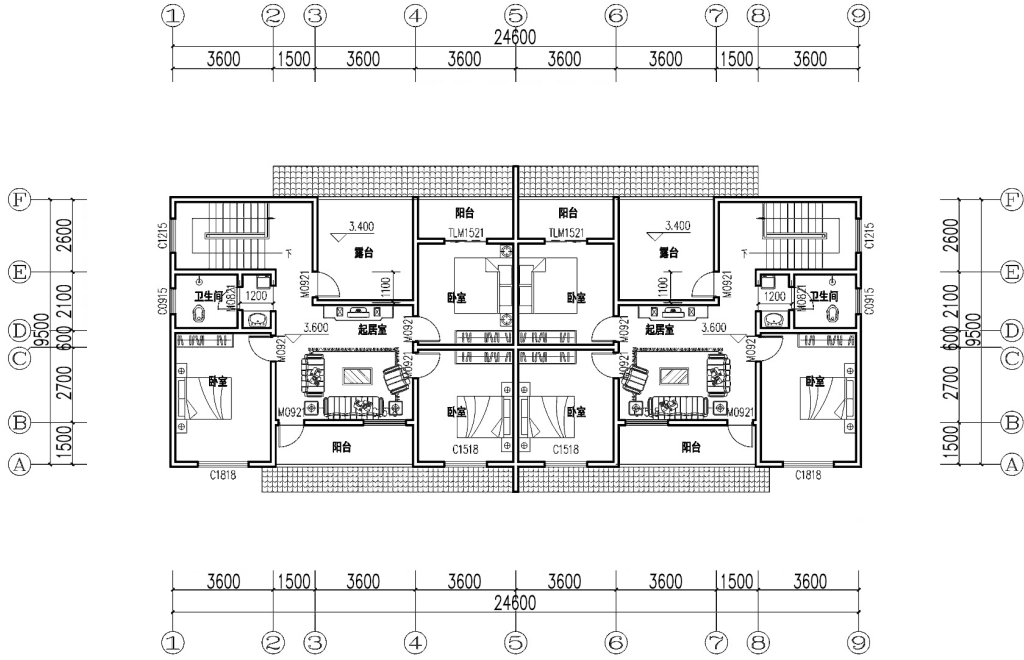
二层平面图
