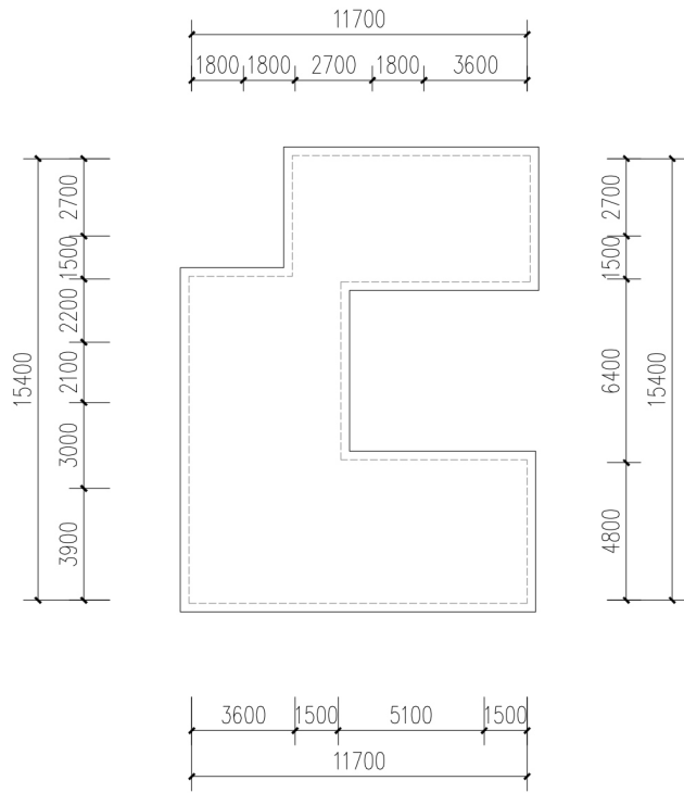
屋顶平面图
