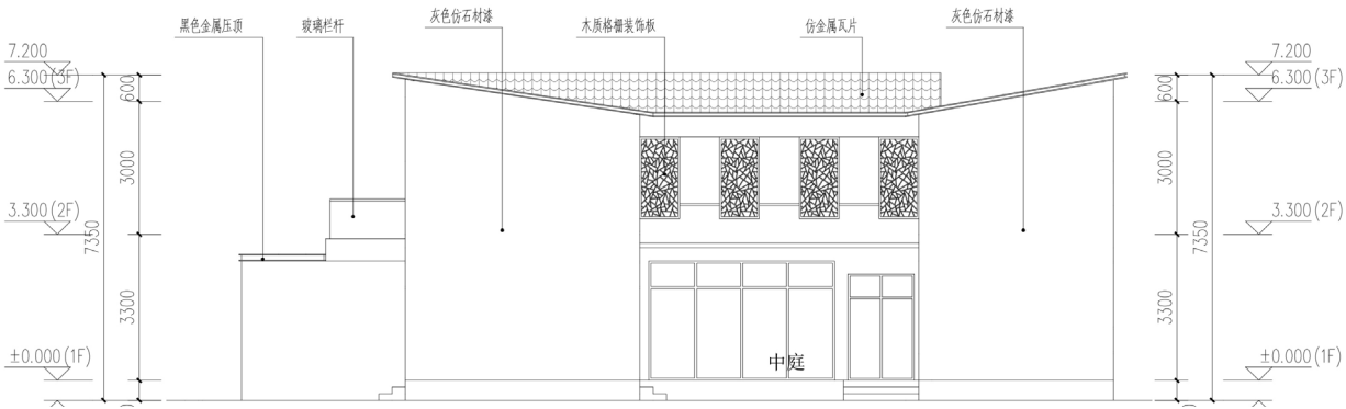
东立面图
