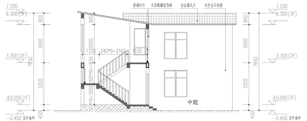
1-1 剖面图
