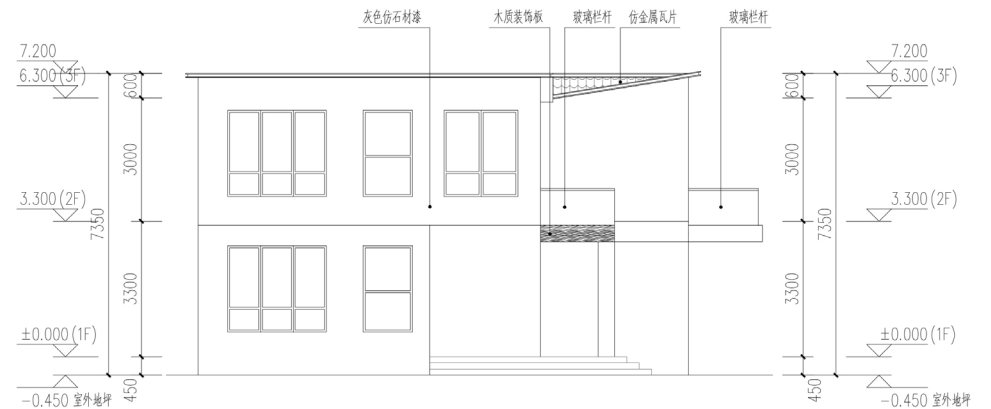
北立面图
