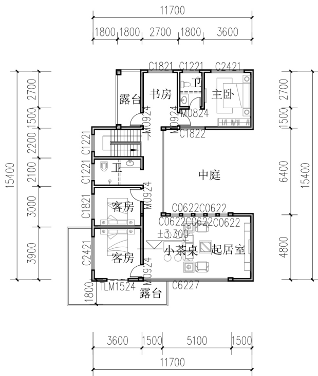
二层平面图
