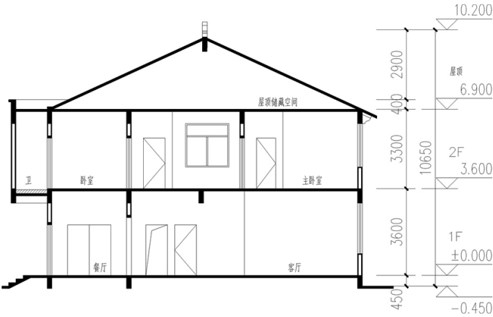
剖面图
