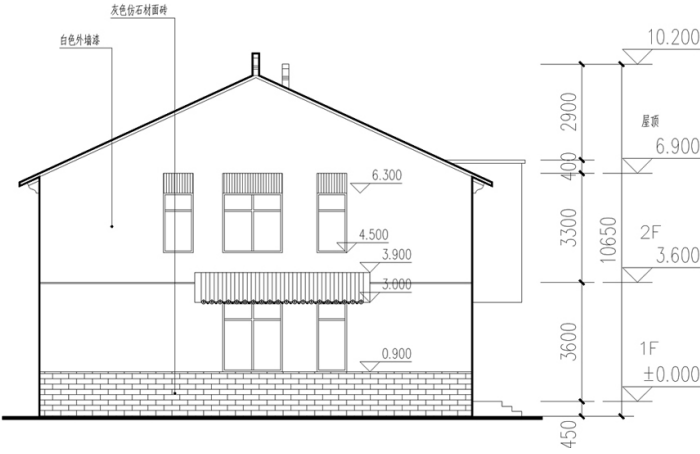
西立面图
