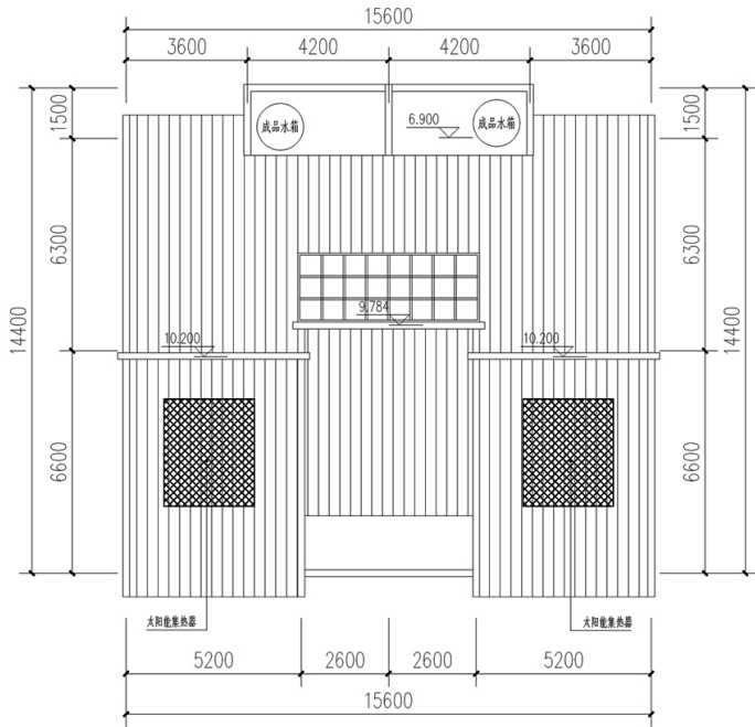
屋顶平面图
