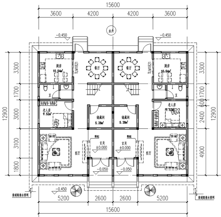
一层平面图
