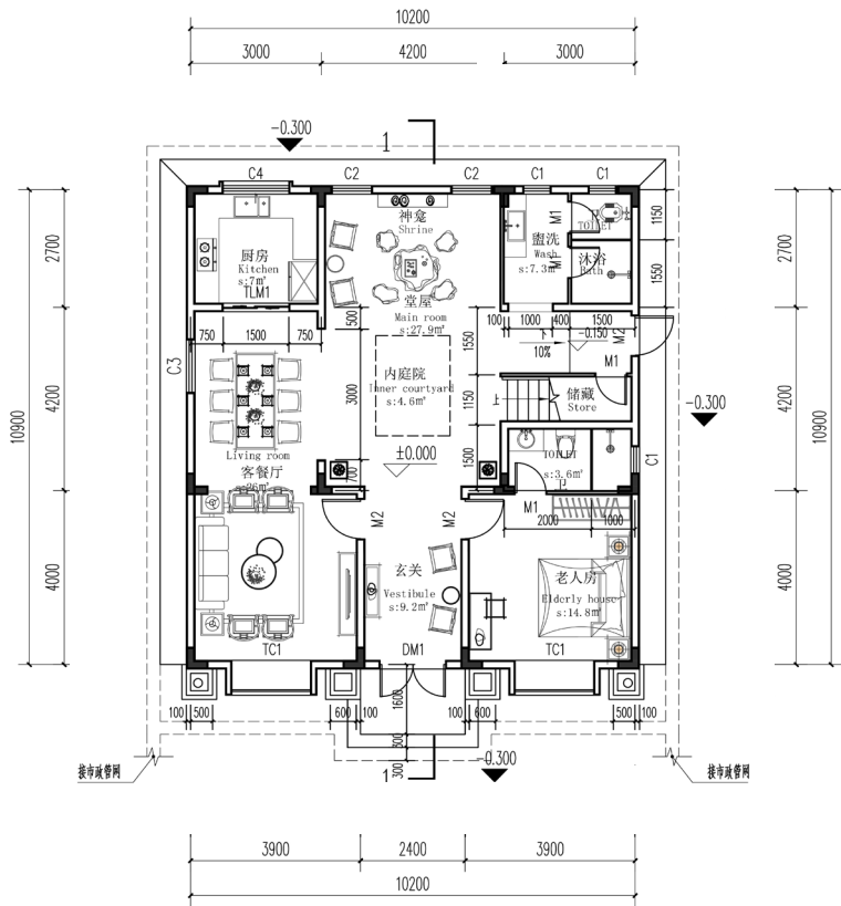
一层平面图
