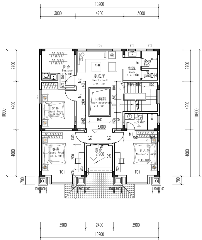
二层平面图
