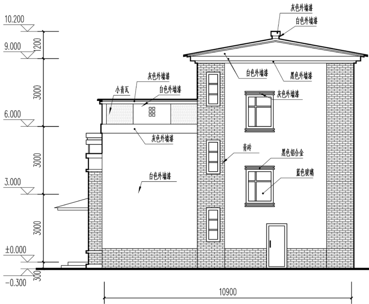
侧立面图
