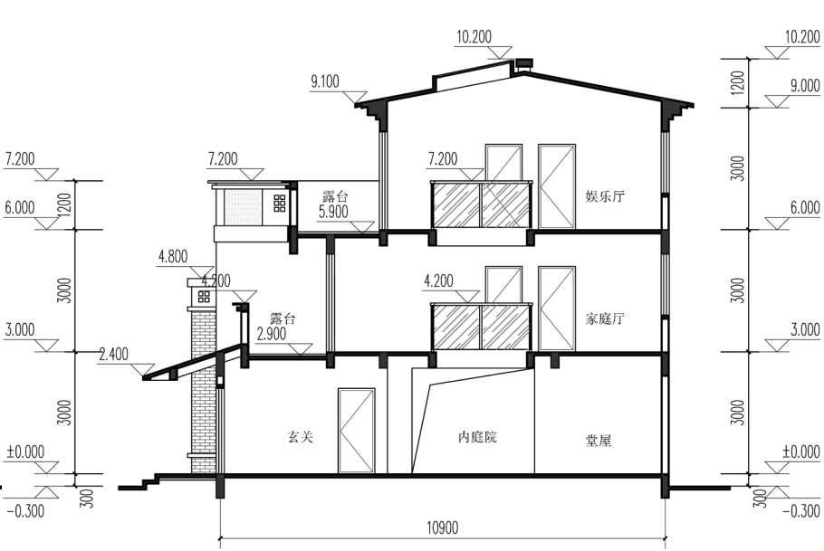
剖面图
