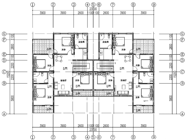
二层平面图
