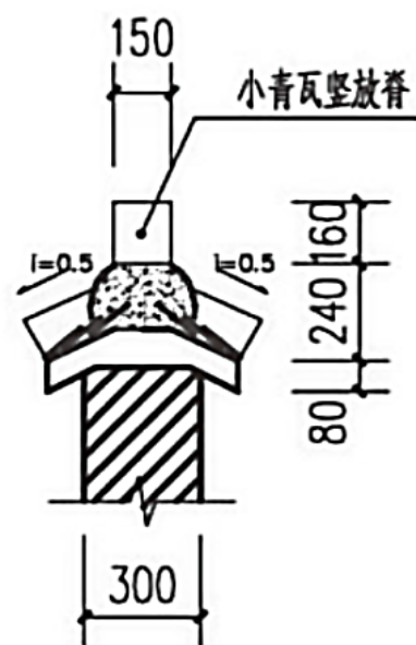
a-a 剖面图
