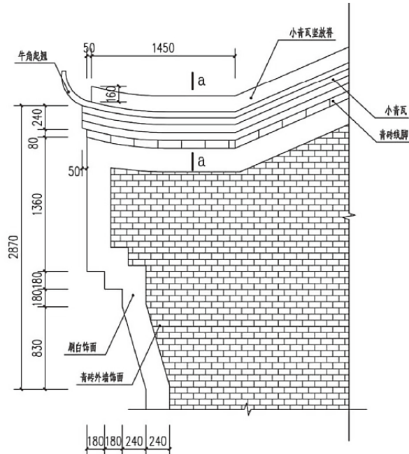
山字形封火山墙墙头大样图
