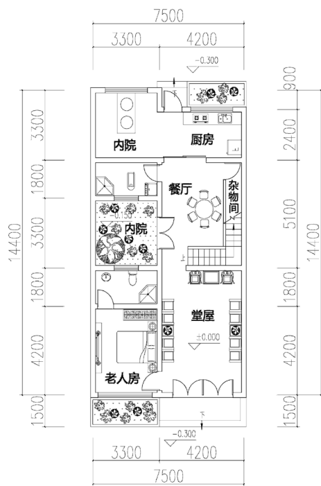
一层平面图
