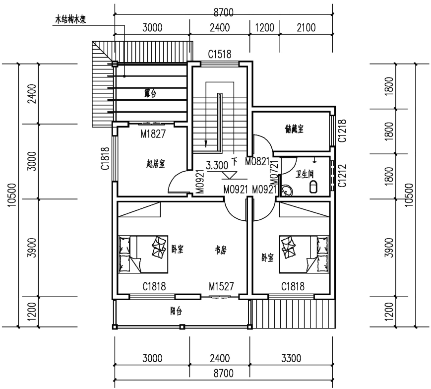
二层平面图
