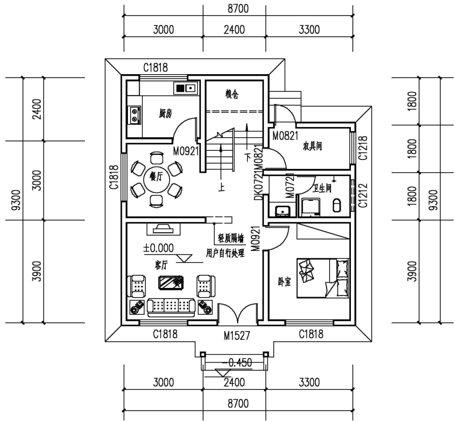
一层平面图
