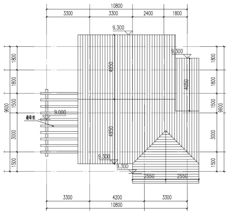
屋顶平面图
