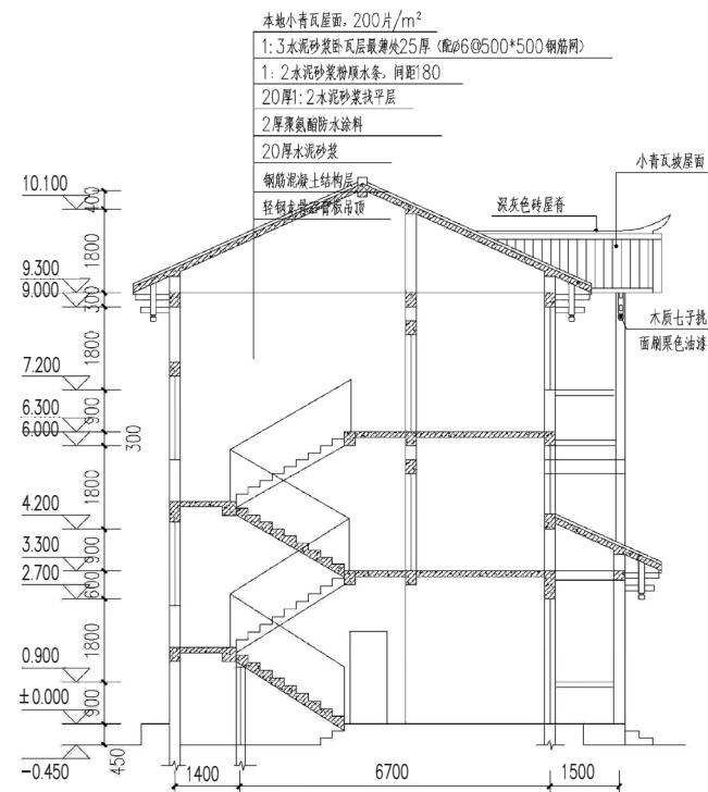
剖面图
