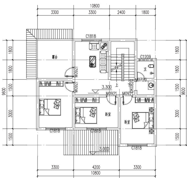
二层平面图
