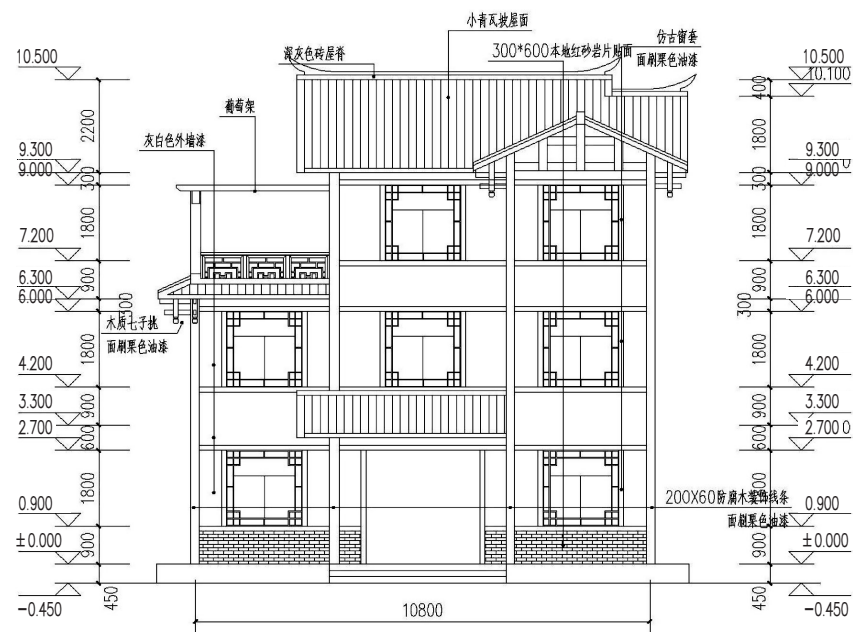
正立面图
