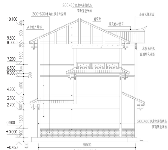
侧立面图
