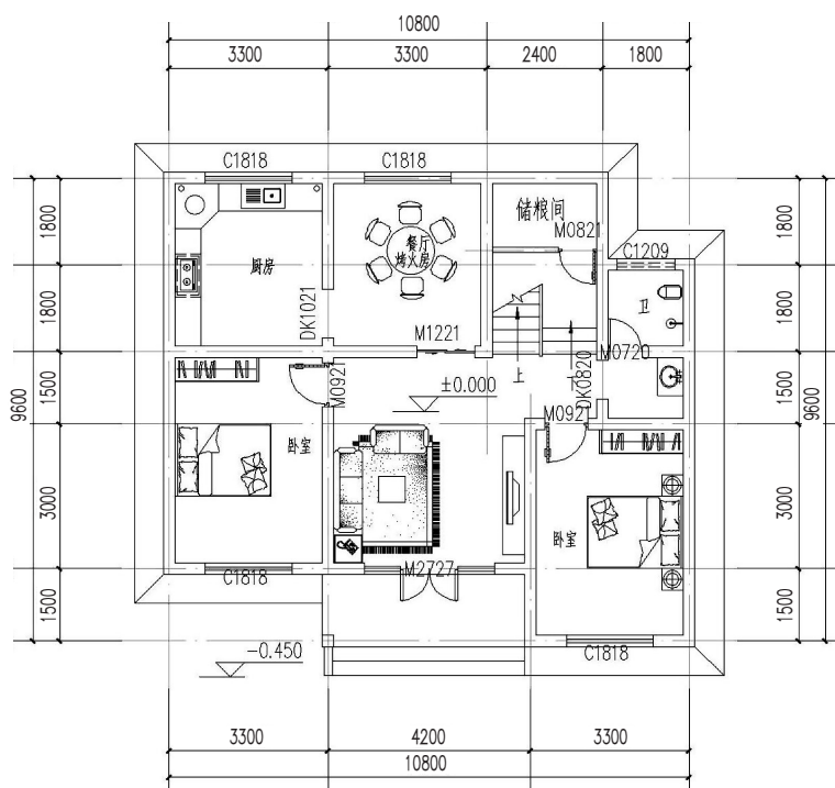
一层平面图
