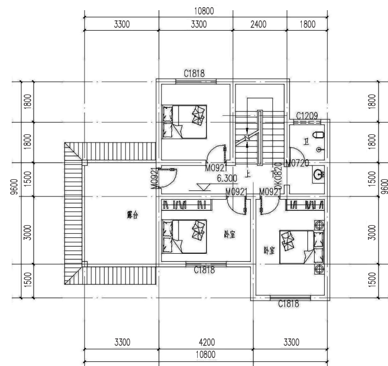
三层平面图
