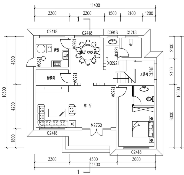
一层平面图
