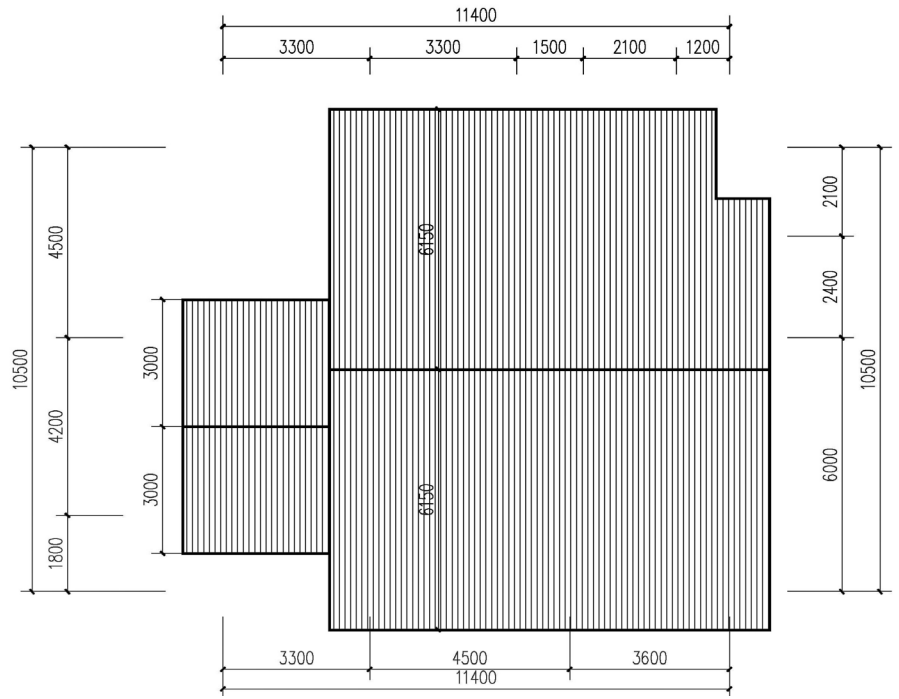
屋顶平面图
