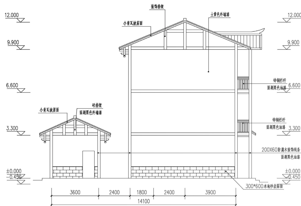
侧立面图
