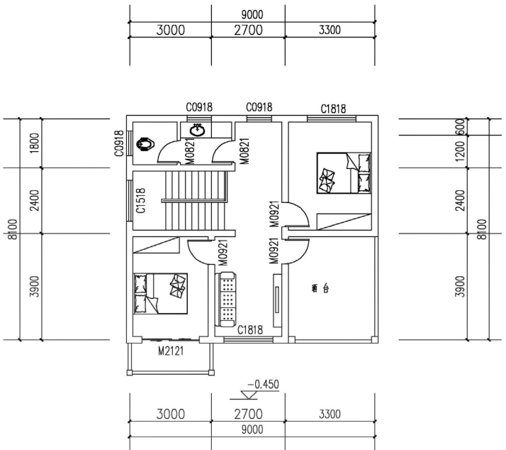
三层平面图
