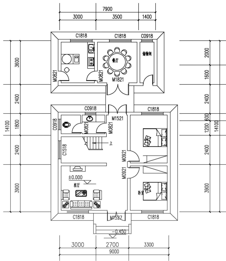
一层平面图
