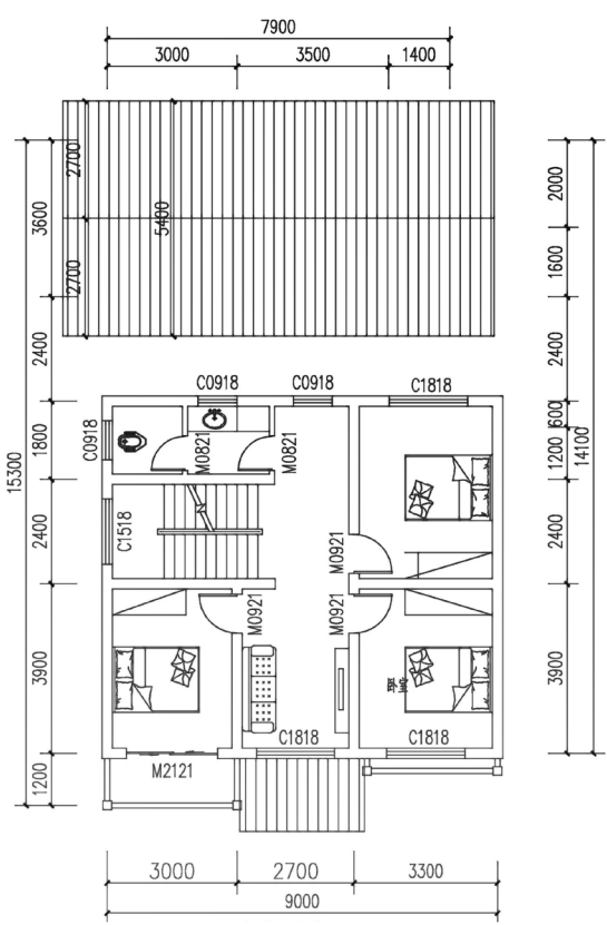
二层平面图
