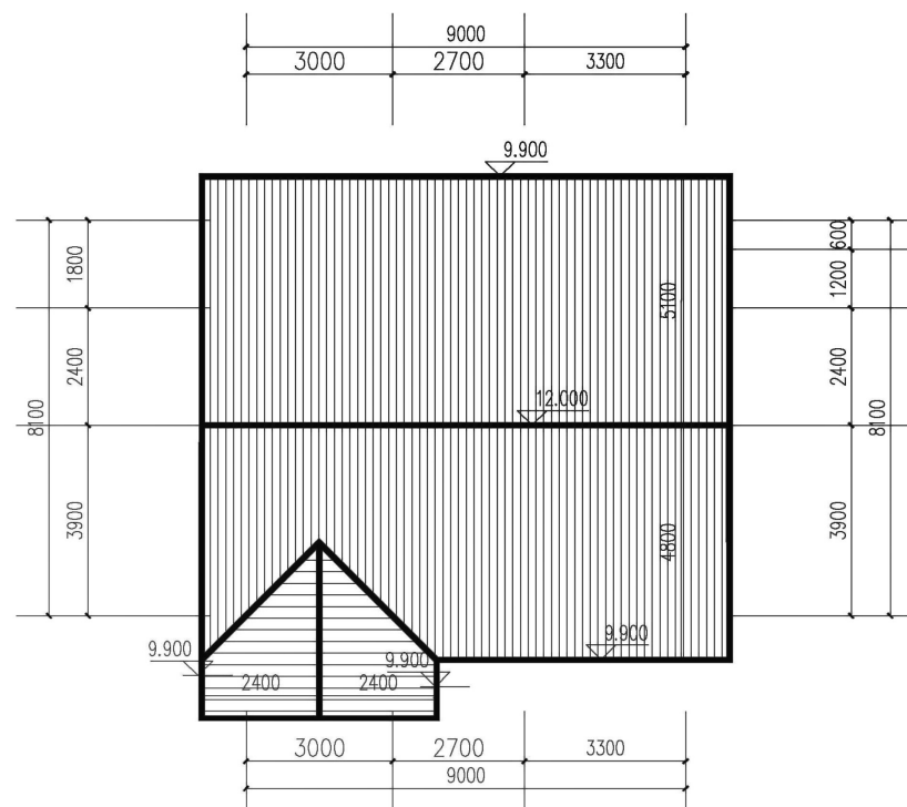
屋顶平面图
