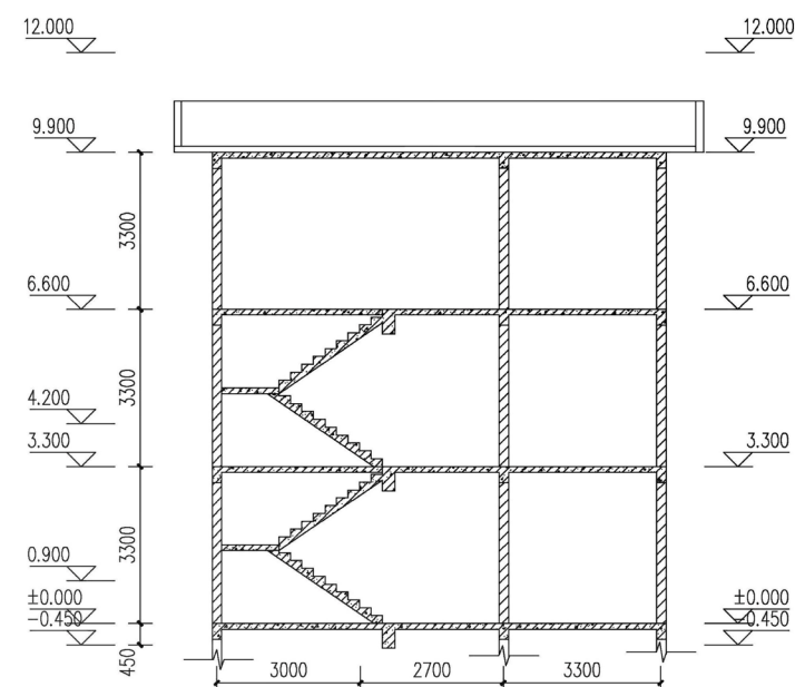
剖面图
