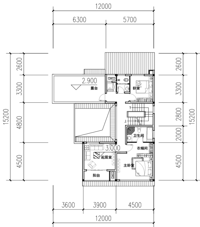
二层平面图
