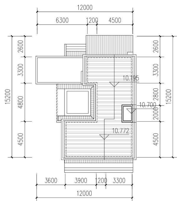
屋顶平面图
