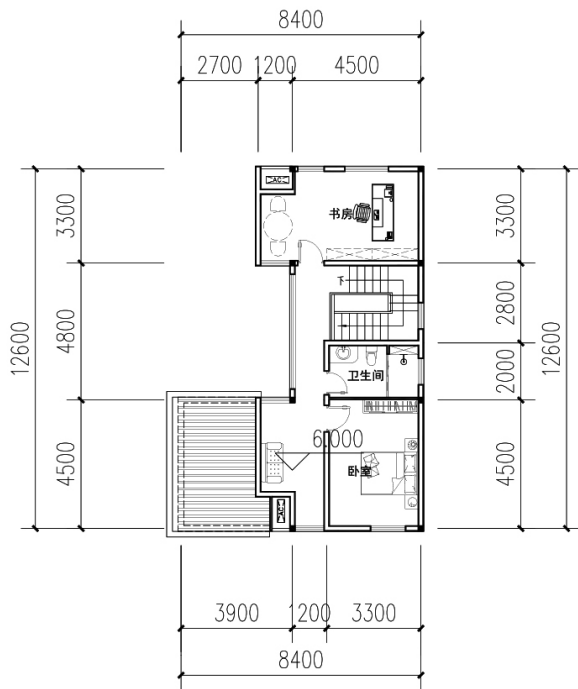
三层平面图
