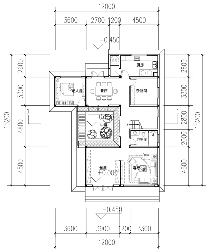
一层平面图
