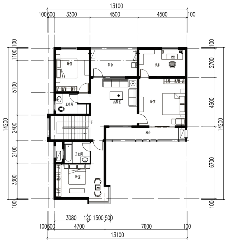
二层平面图
