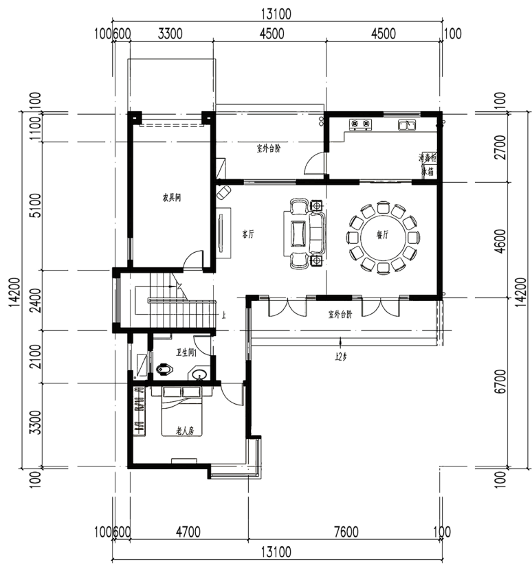
一层平面图
