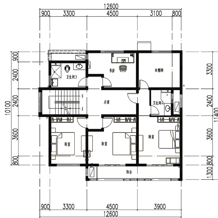
二层平面图
