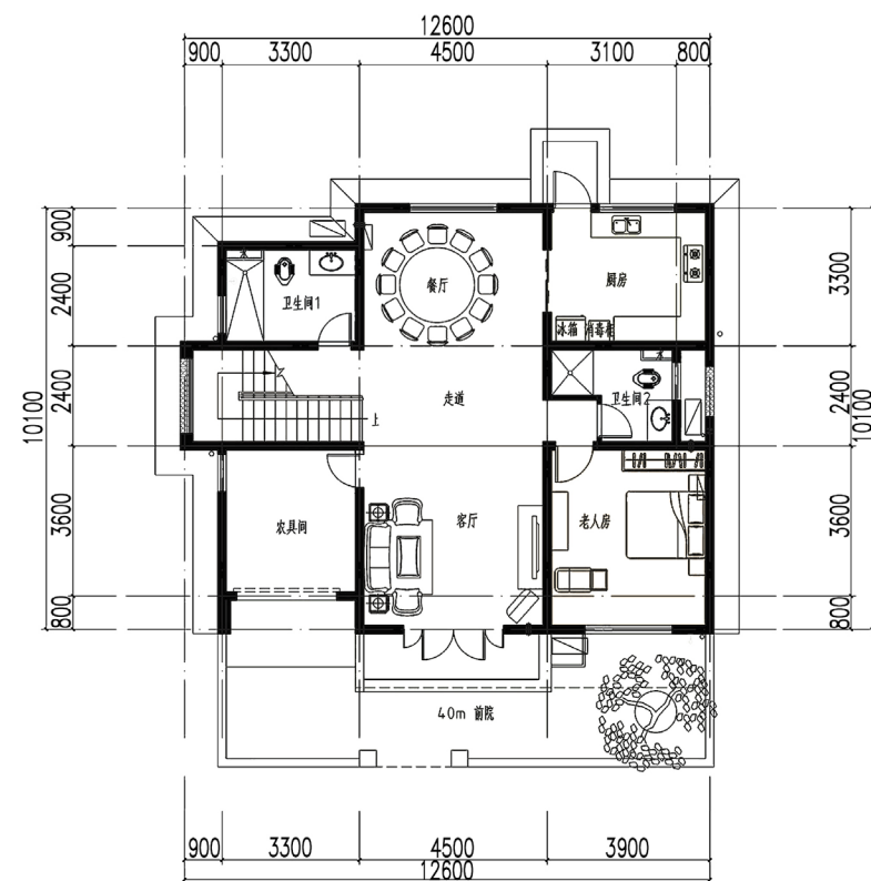
一层平面图
