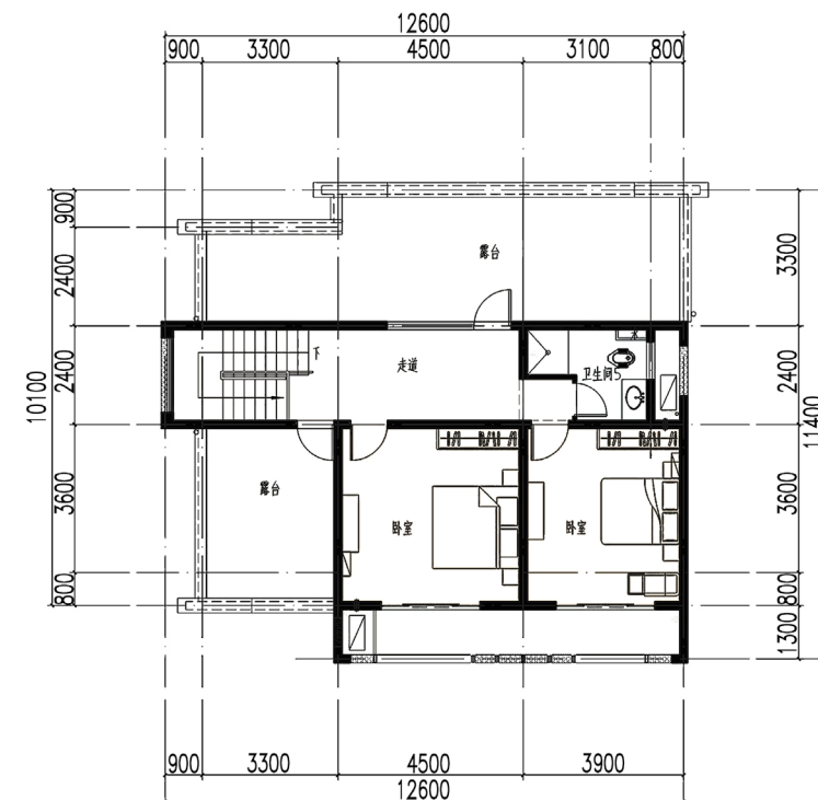
三层平面图
