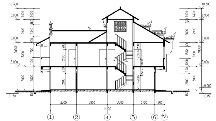
剖面图
