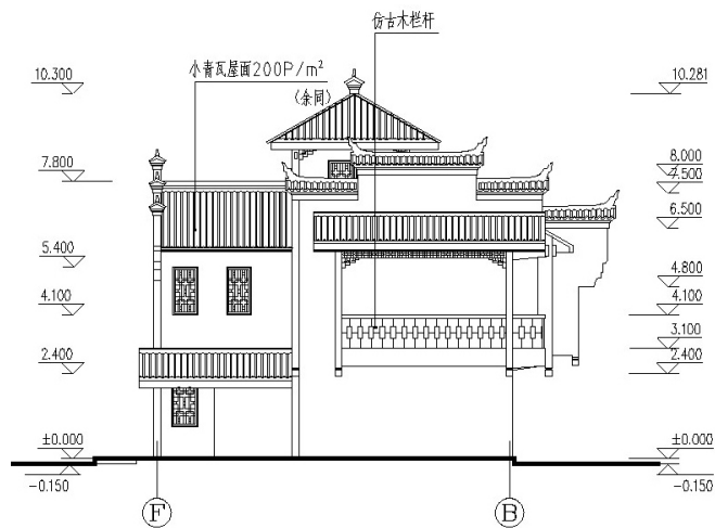
西立面图
