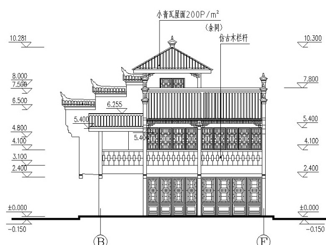
东立面图
