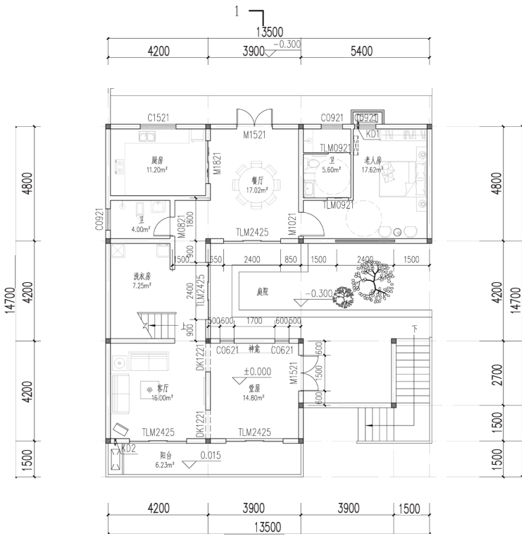
二层平面图
