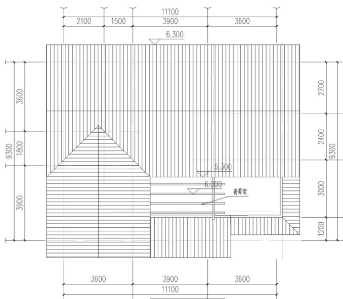
屋顶平面
