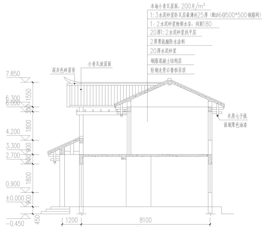
剖面图
