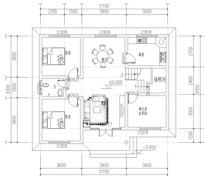
一层平面图
