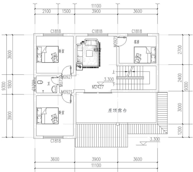
二层平面图
