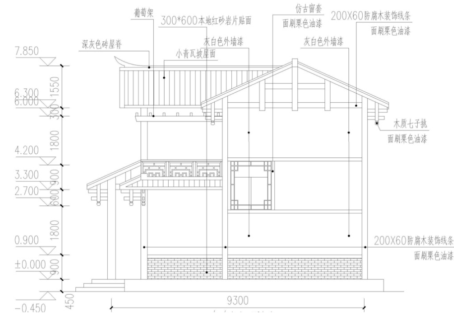
侧立面图
