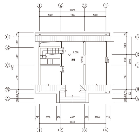
屋顶层平面图
