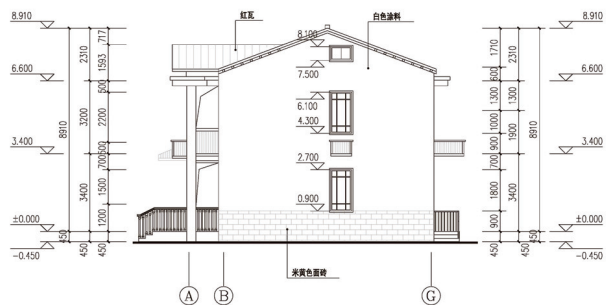
东立面
