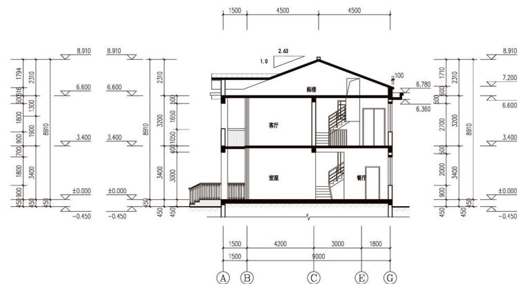
1-1 剖面图
