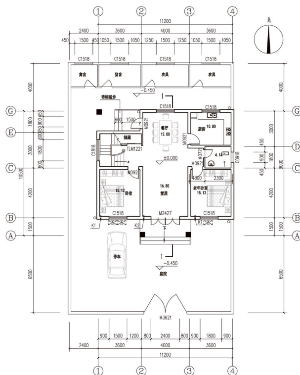
一层平面图
