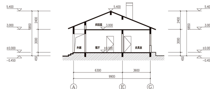
1-1 剖面图
