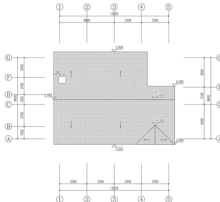
屋顶平面图
